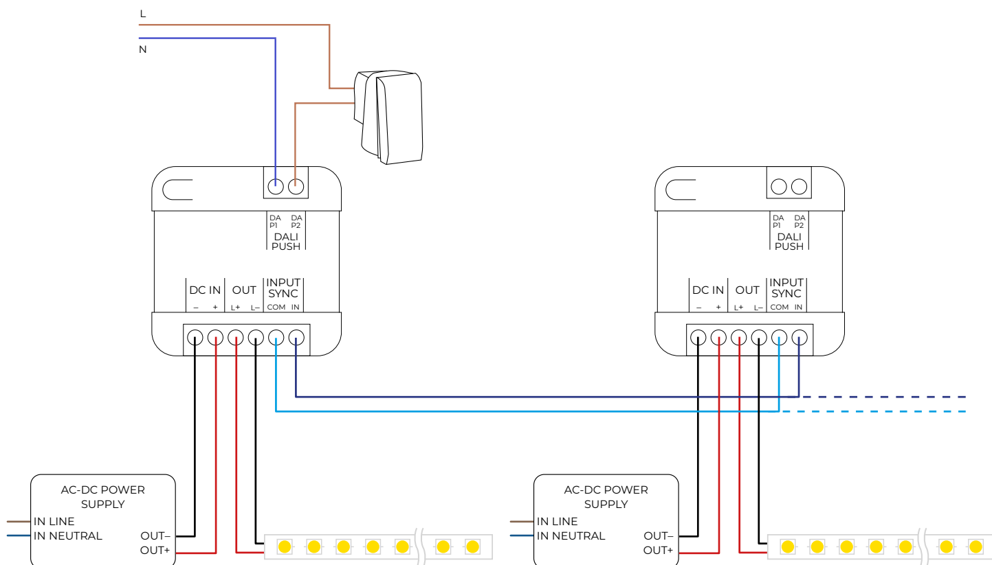
FIG. 11 - collegamento slave a DALI2-CV-M2 con ingresso PULSANTE
