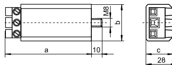
PC casing – K D20
