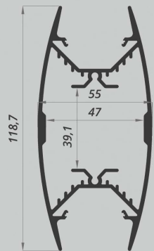
Profilo dissipatore led in alluminio per sospensione (Consigliato l'utilizzo con strip LED fino a 50 W/m)
